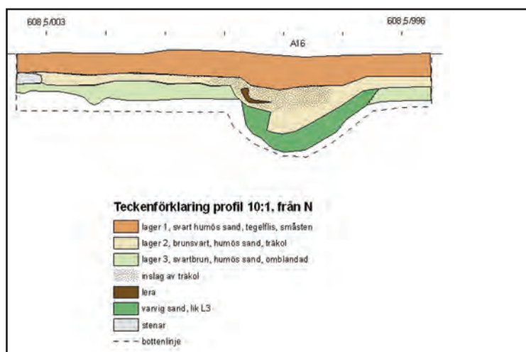
FIGUR 30. Profil ugnen A 16 (Profil 10:1).
