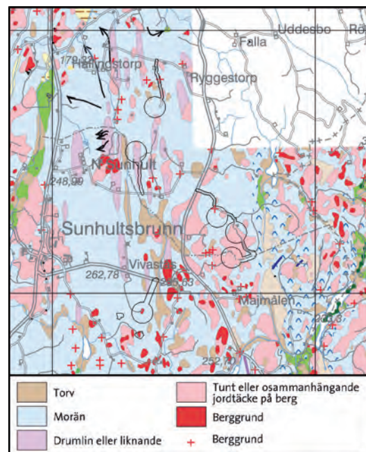
FIGUR 2. Geologisk karta över UO, med uppställningsplatserna markerade. SGU.
