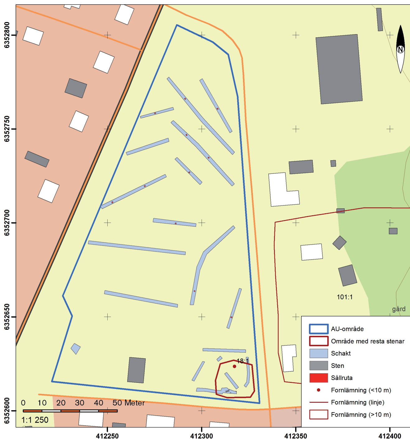
FIGUR 3. Schaktplan. Skala 1:2 000.
