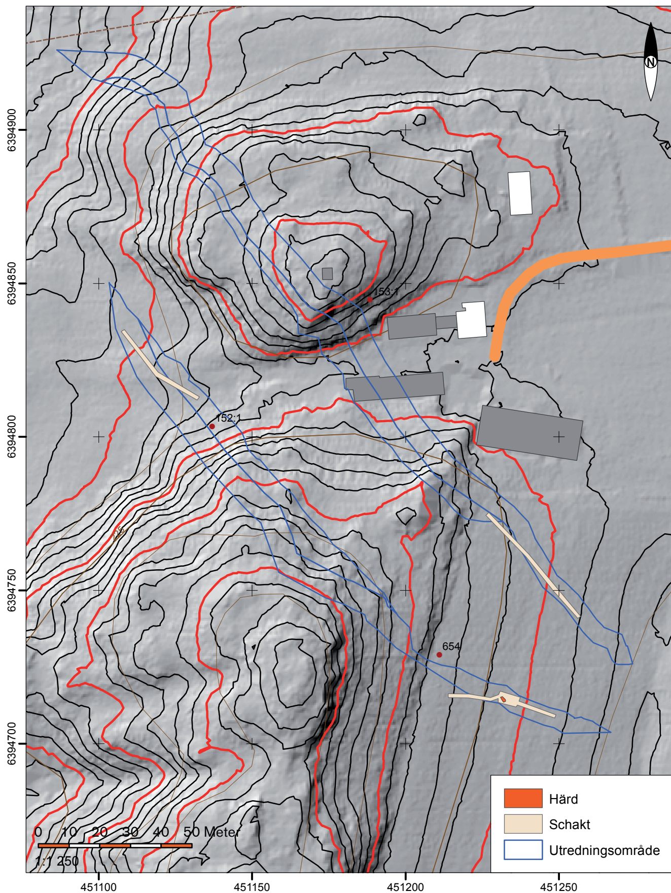
FIGUR 3. Höjdmodell med schakten och utredningsområden. Skala 1:1 250.
