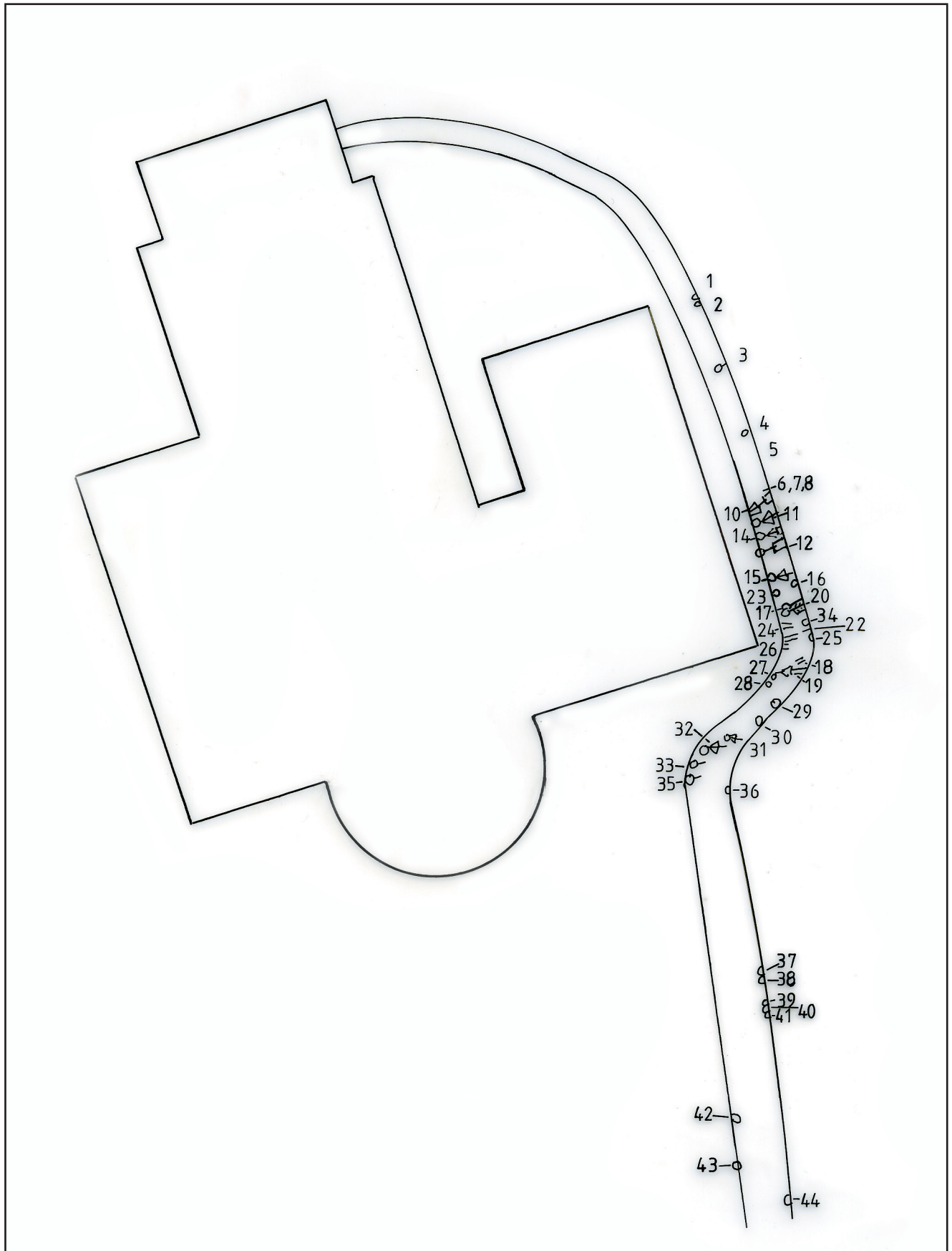
Plan över schaktets dragning och anläggningarna. Renritad av Björn Varenius, 1985. Skala: 1:200.
