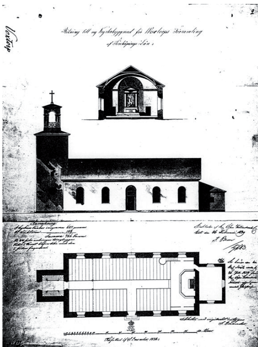
Kyrkan byggdes 1841-43 efter ritningar av byggmästaren Berndtsson. Denna ritning är från 1838.
