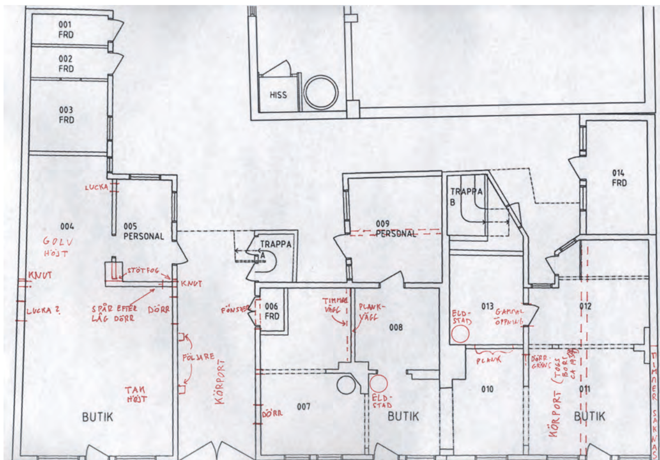
Planritning över bottenvåningarna till Smedjegatan 11 (den till vänster liggande 2/3) och Smedjegatan 13 (den till höger liggande 1/3). De röda kommentarerna preciserar byggnadsarkeologiska iakttagelser. De dendrokronologiska proven togs i bottenvåningens gatufasad.
