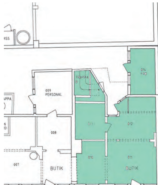
Smedjegatan 11, bottenvåningen, grönmarkerad.
