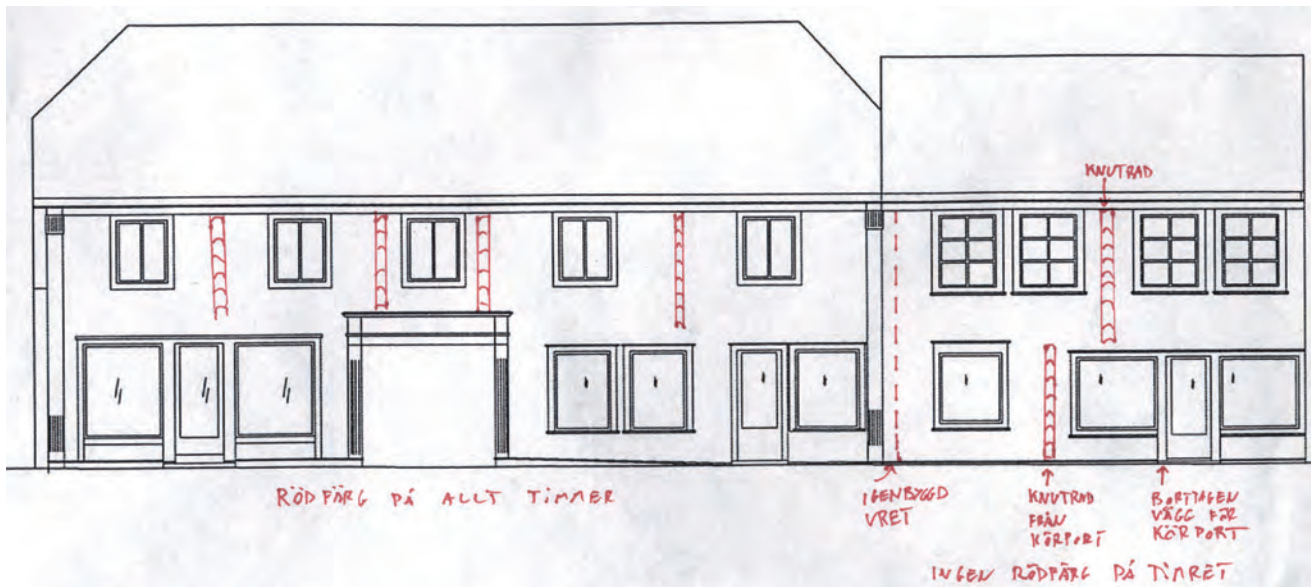
Detaljanalys av gatufasadernas timmerstommar.
