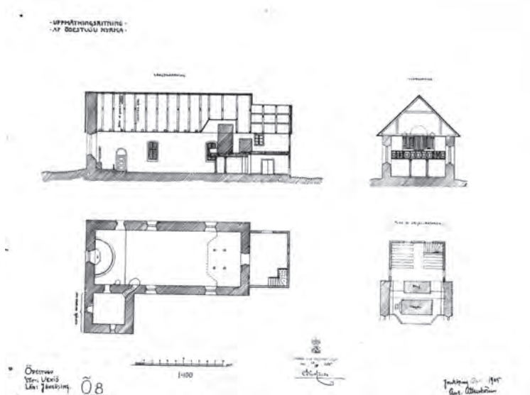
Uppmåtningsritningar från 1905 av arkitekt August Atterström.
