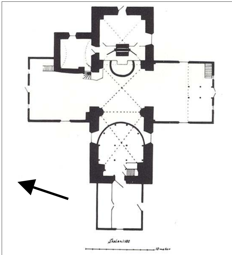
Plan över Askeryds kyrka upprättad av K D Andersson. Ritning från Kilstrom, 1991.
