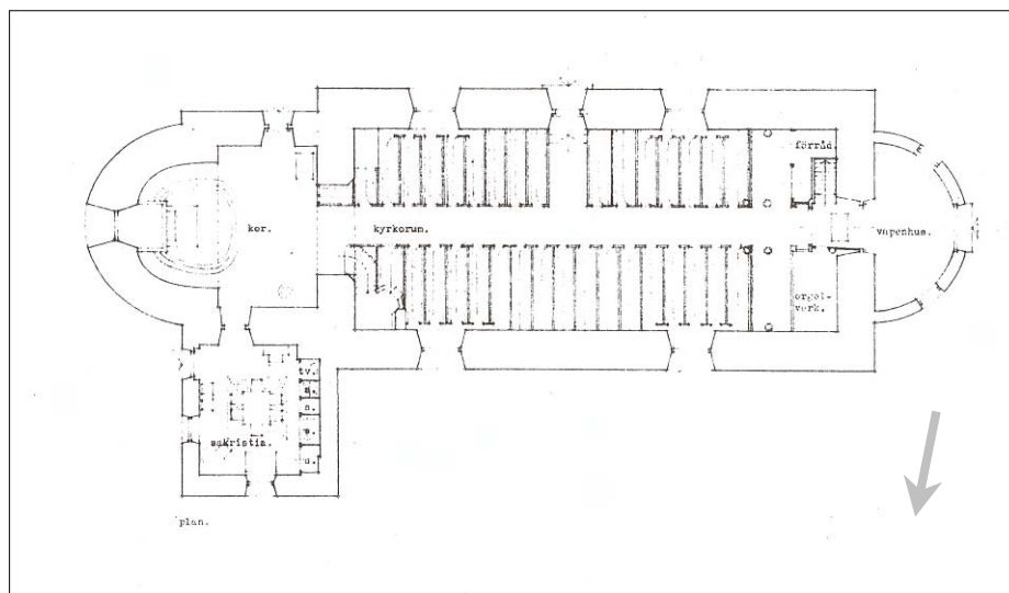
Plan över Bredestad kyrka, förslagsritning från Johannes Dahls arkitektfirma 1961 inför restaurering. Ändringar genomfördes i stort sett enligt ritningarna. Ritning från Länsstyrelsen i Jönköpings läns arkiv.
