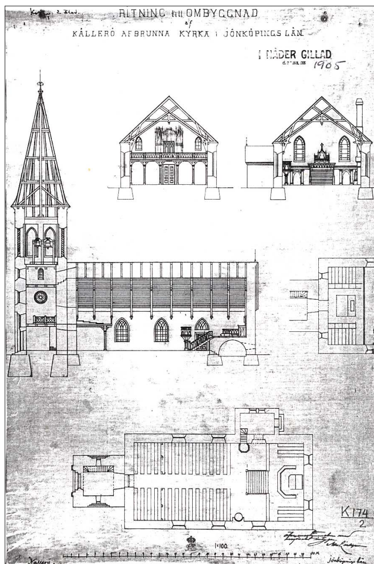
Ritningar till den nya kyrkan upprättade efter branden 1904
