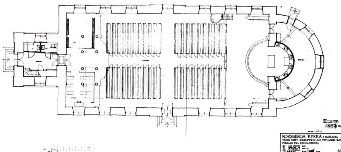
Restaureringsritning upprättad av arkitekt Lars Löfstedt. 1980.
