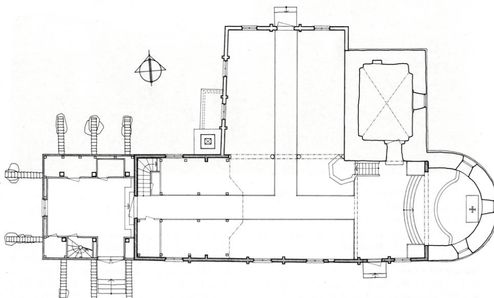
Plan över Vireda kyrka, utförd av G Wirén, 1980.
