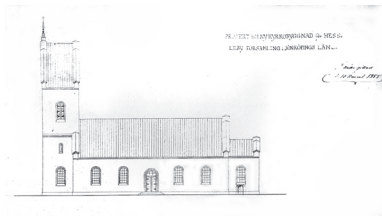
Scholanders plan respektive fasadritning för Hässleby kyrka.
