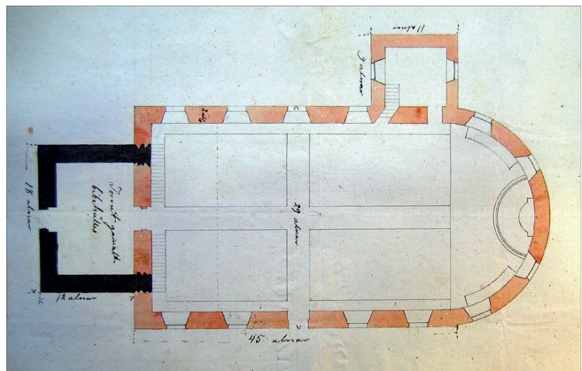
Plan Ingatorps kyrka, RA.
