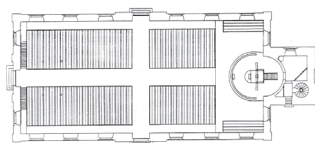
Uppmättningsritning Adelövs ka
