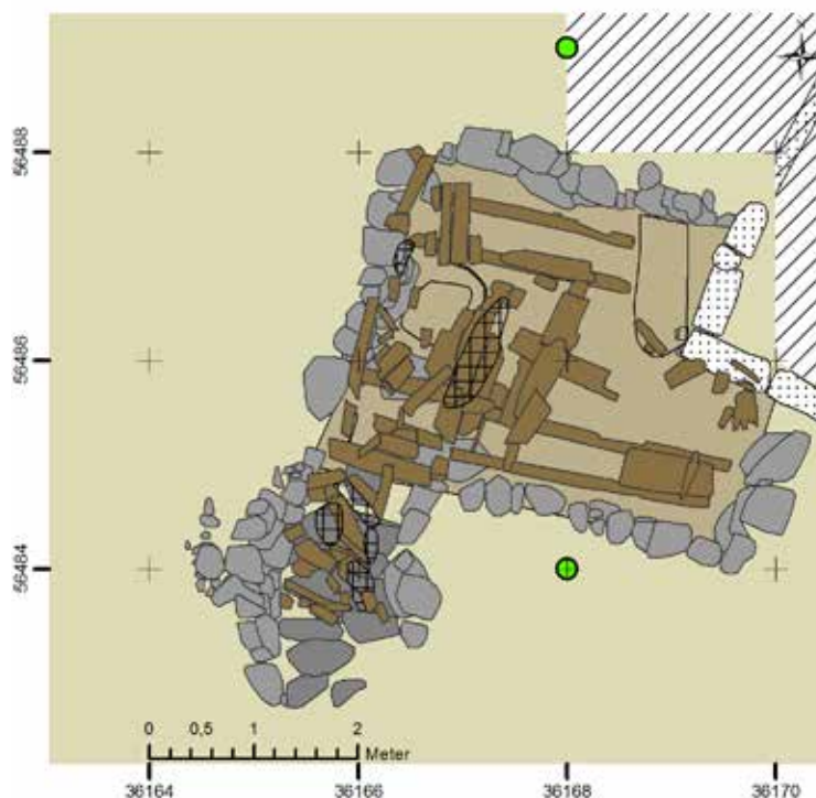
Figur 40. Ritning över stenkällaren A 74. Gröna punkter markerar sektionsritning (se figur 42). Vitmarkerade ytor i övre högra hörnet är dels en sentida mur (prickad yta) och tidigare urschaktad yta (streckad).
