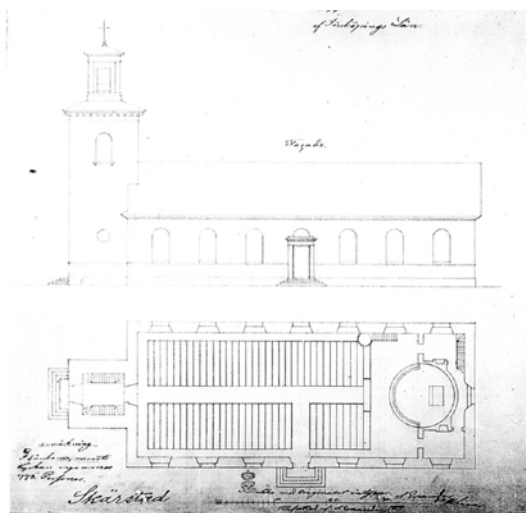
Ovan: Arkitekt Samuel Enanders ritning för Skärstads kyrka 1817. ATA.
