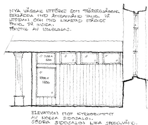
Ovan: Ritning av 2003 års läktarunderbyggnad. Fönstren åstadkom både ljus in till underbyggnaden och samtidigt en visuell kontakt ut mot kyrkorummet. Ritning av Ingvar Selse, Arkitekthuset. Till vänster: Läktarunderbyggnad från 2003.
